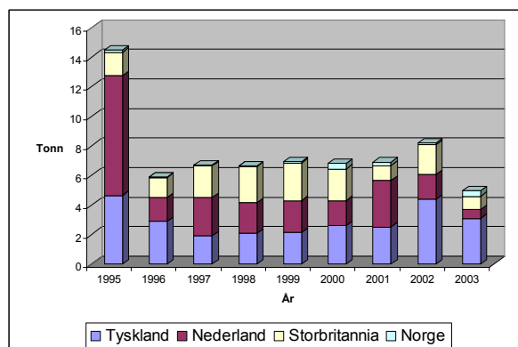
Figur 5.41 Utslipp av kvikksølv fra landbasert virksomhet (direkte tilførsler (avløp og industri) og elvetilførsler) til Nordsjøen fordelt på land (kilde OSPAR 2001, 2004c, 2005b). Data fra Danmark er ikke rapportert.
