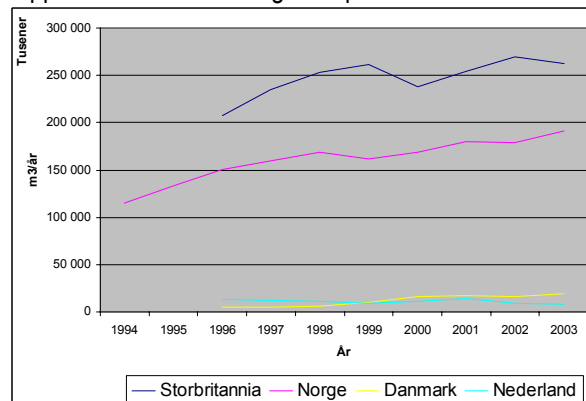
Figur 5.12 Utslippsmengder av produsert vann og fortreningsvann til Nordsjøen fordelt på land (OSPAR 2005). Utslippsmengden for Norge gjelder hele norsk sektor, og ikke kun for de fire regionene.
