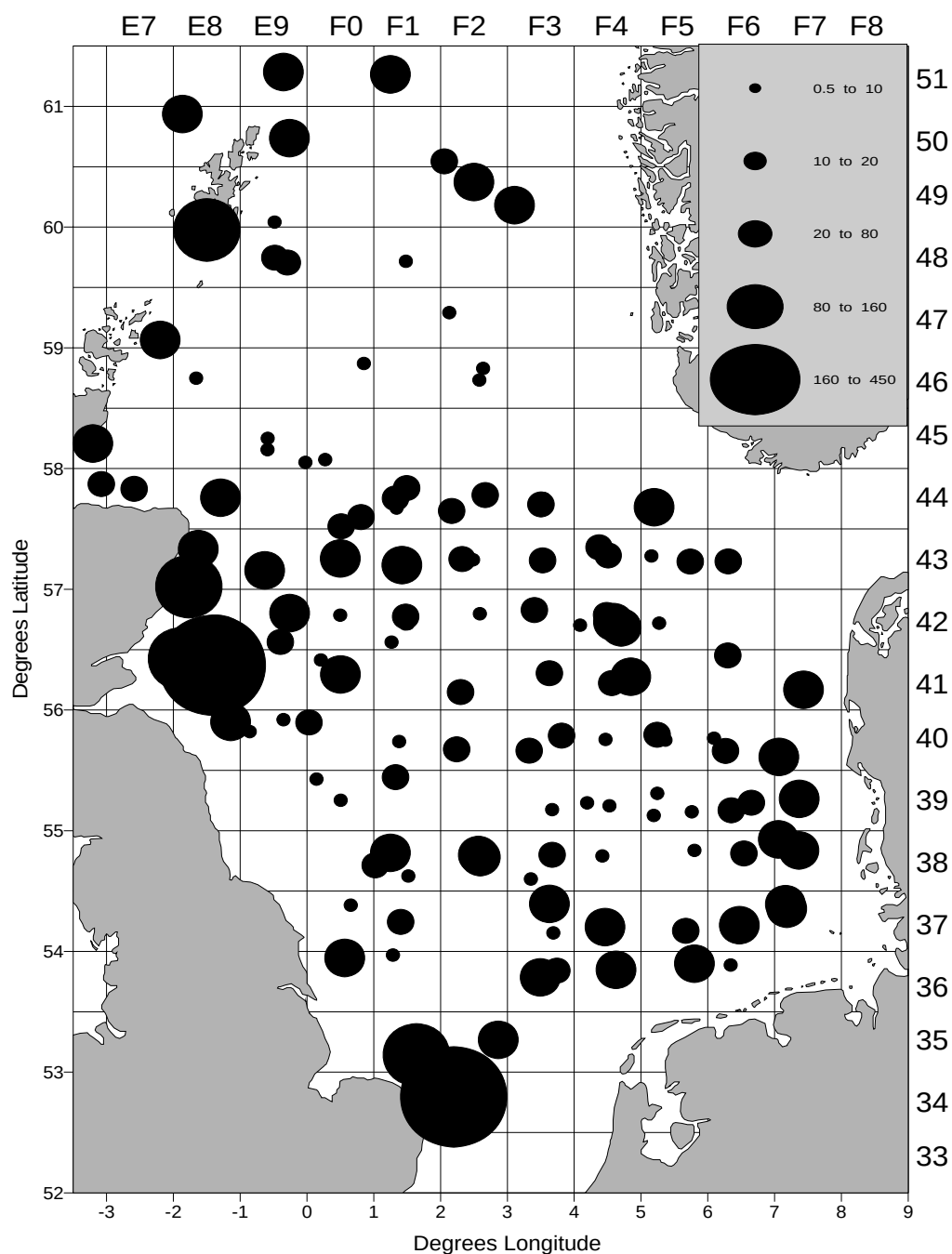
Figur 3.22. Kartet viser hvor mange milligram dyresamfunnet oppå sedimentet på 1 m 2 havbunn øker per dag. Figuren er hentet fra MAFCONS hjemmeside http://www.mafcons.org/
