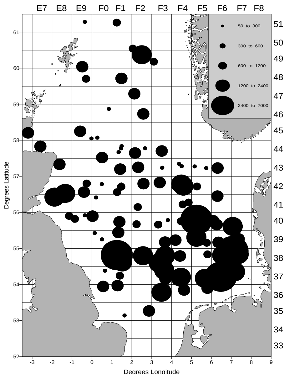
Figur 3.23. Kartet viser hvor mange milligram dyresamfunnet av gravende dyr på 1 m 2 havbunn øker per dag. Figuren er hentet fra MAFCONS hjemmeside ( http://www.mafcons.org/ ).
