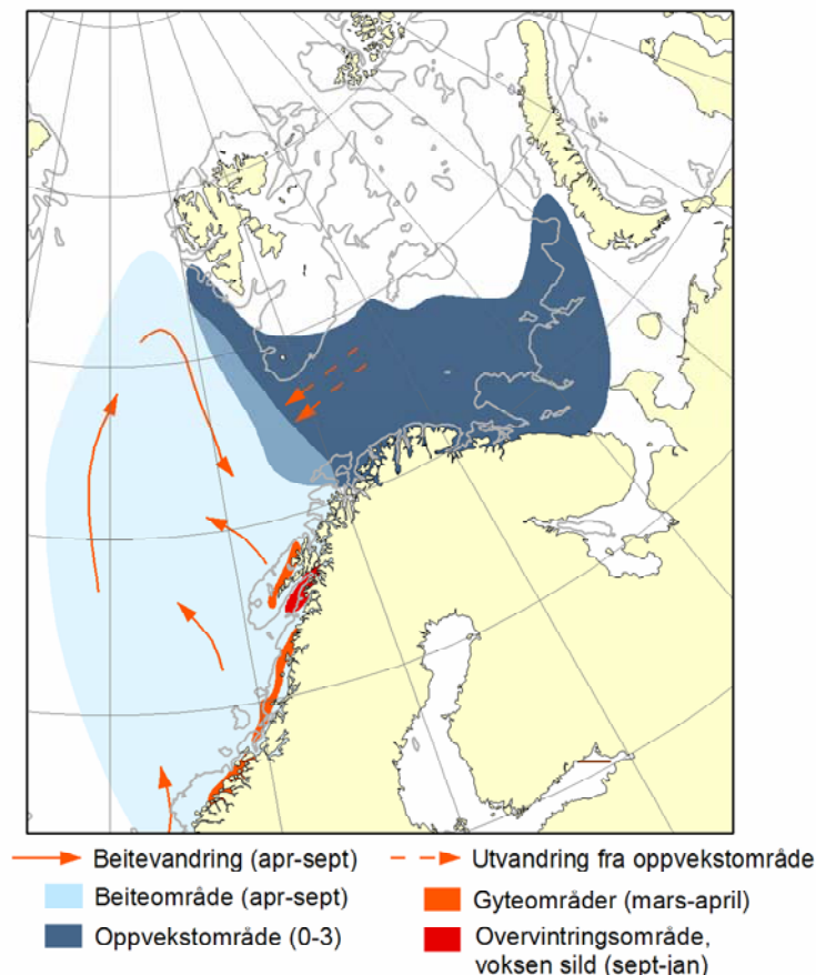
Figur 3.15. Fordelingsmønster hos norsk vårgytende sild.
