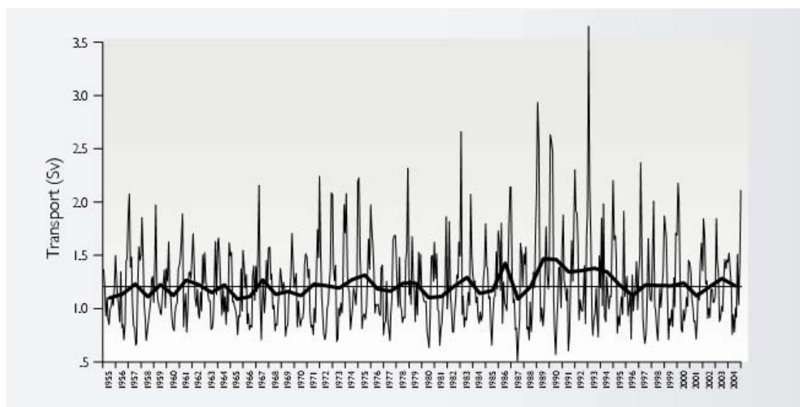
Figur 4.1. Tidsserier (1955–2004) av modellert årsmidlet (tykk strek) og månedsmidlet transport av atlantisk vann til den nordlige og sentrale Nordsjøen sørover mellom Orknøyene og Utsira. 1 Sv = 10^6 \text{ m}^3 \text{ s}^{-1} .
